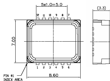
SCA830外形寸法図
