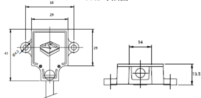
SCA121T-D03/05/07 外形寸法図
