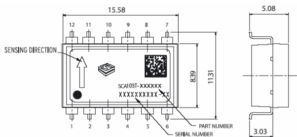
SCA61T/100T/103T外形寸法図
